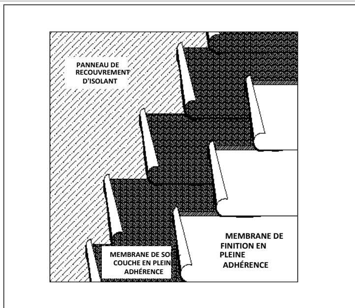
Figure 3 : Détail de l'installation du système de membrane de toiture de bitume modifié au SBS
