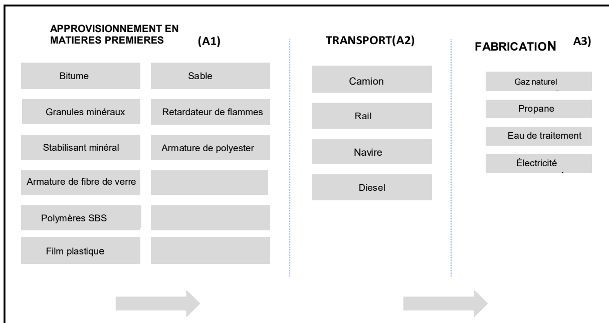
Figure 1 : Aperçu du processus de production
