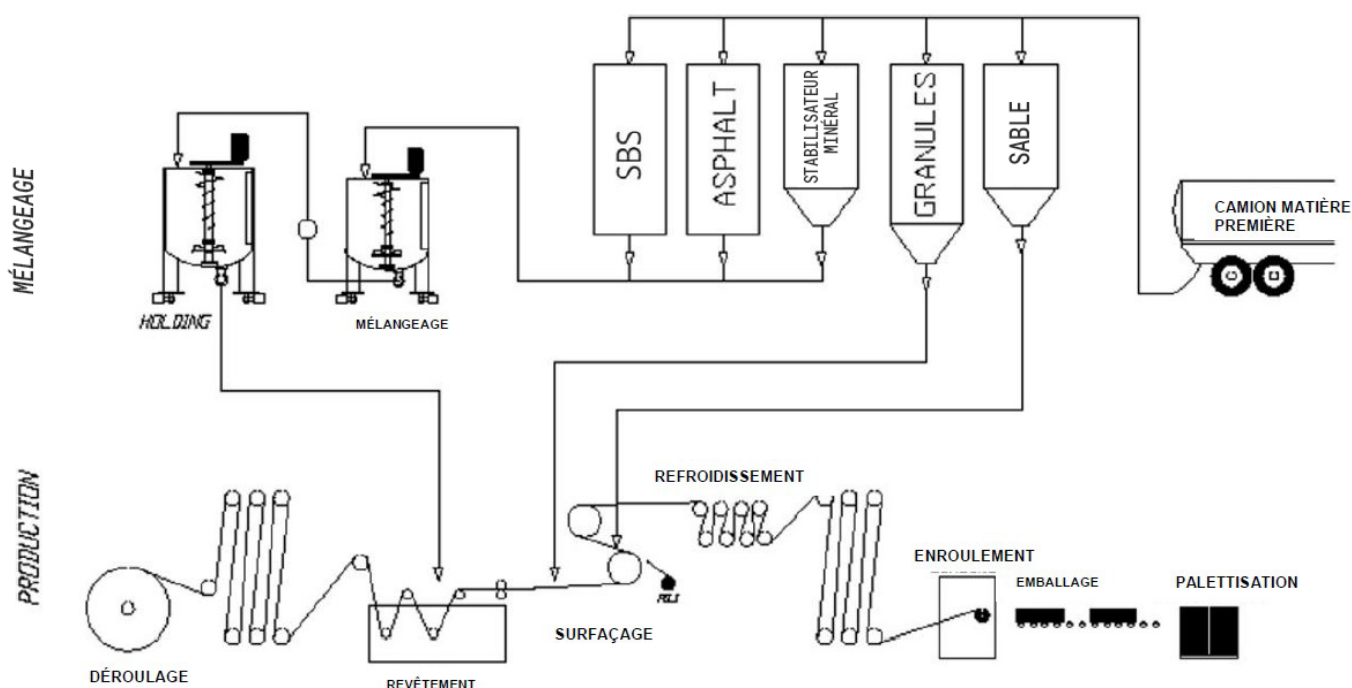
Figure 2 : Diagramme du processus de fabrication des membranes de bitume modifié
